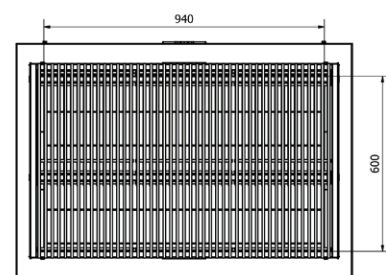
VUE SUPÉRIEURE
