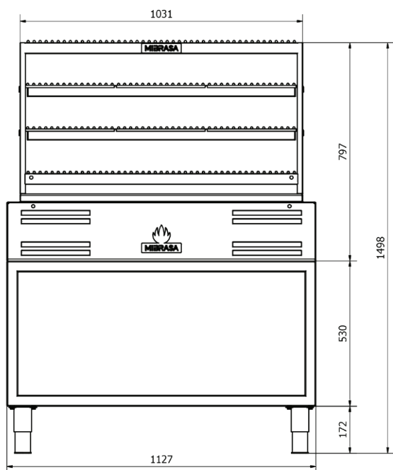
VUE FRONTALE
