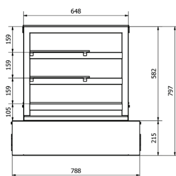
VUE LATÉRALE
