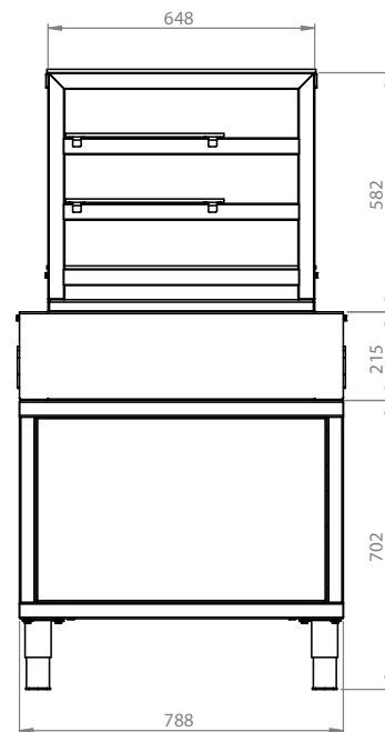
VUE LATÉRALE
