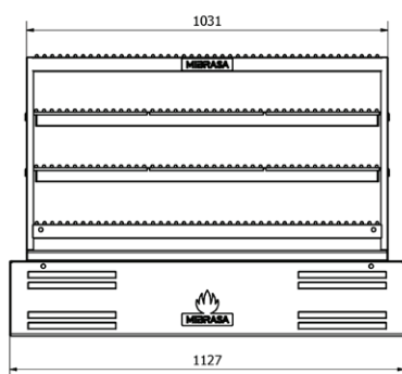
VUE FRONTALE
