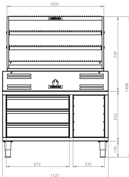
VUE FRONTALE
