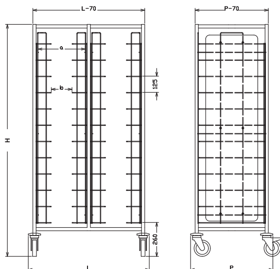
Chariot 2 x 12 niveaux entrée sens largeur (double entrée côte à côte). Vue de face.
